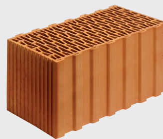
POROTHERM Profi 44 Ti
